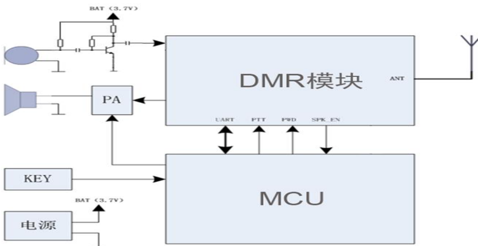
图 1 典型应用电路框图
