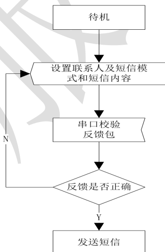
图 3 非确认短信发送流程
