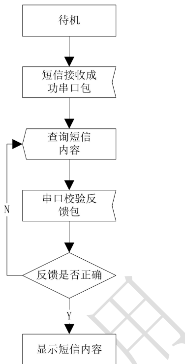
图 4 非确认短信接收流程
