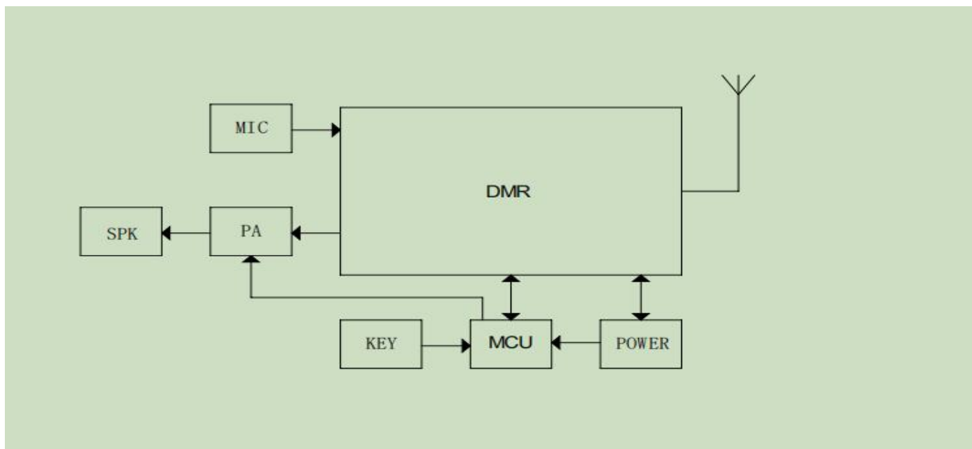
图 1 典型应用电路框图
