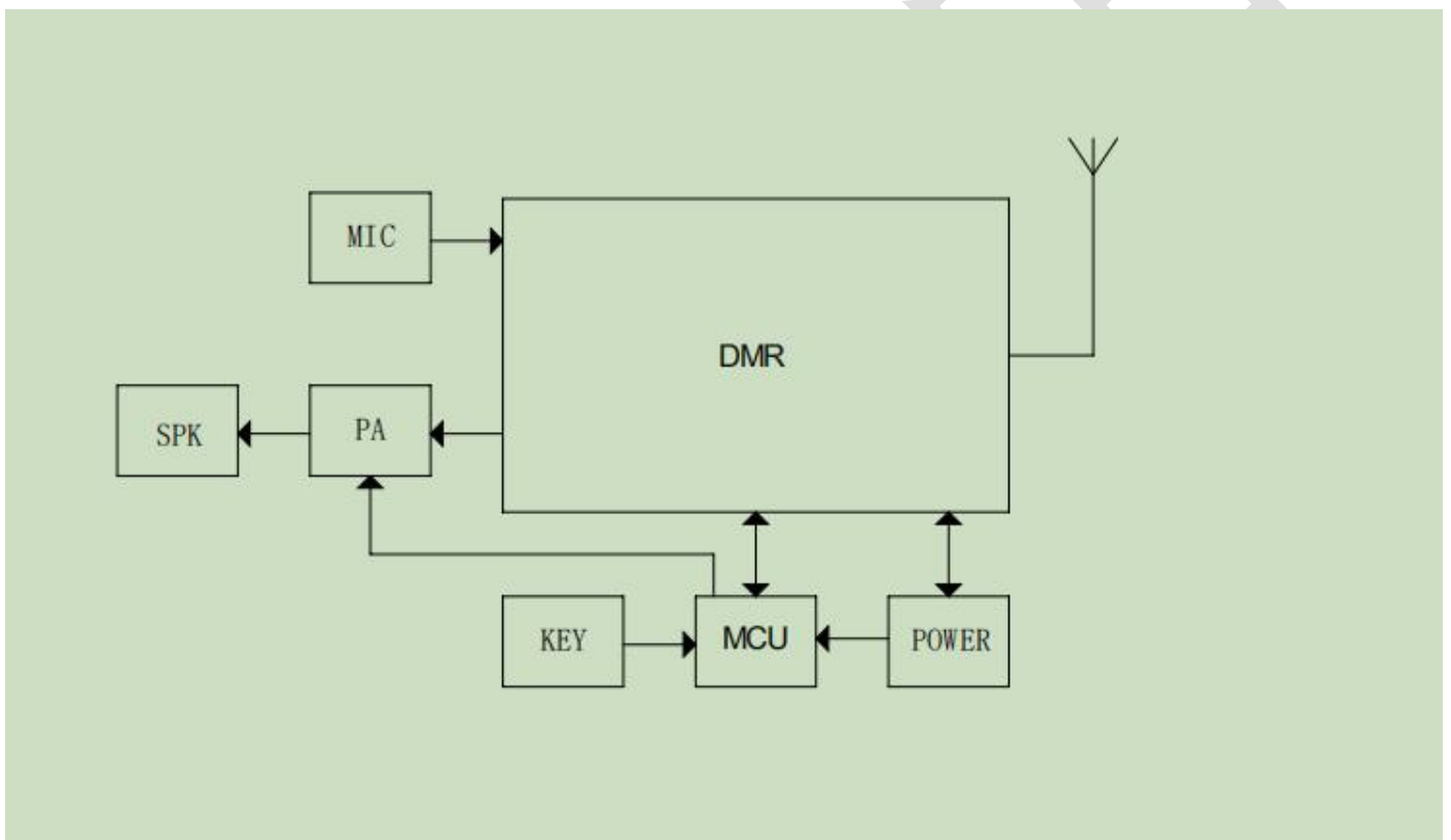
图 1 典型应用电路框图
